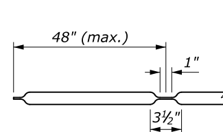
LONGITUDINAL DRAINAGE BAR
